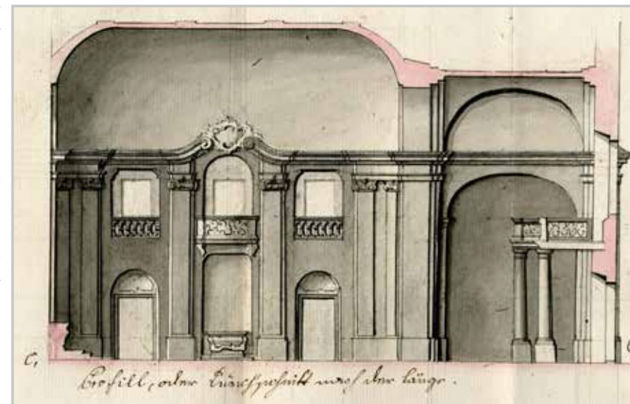
Nerealizovaný návrh: podélný řez svatohorským kostelem
