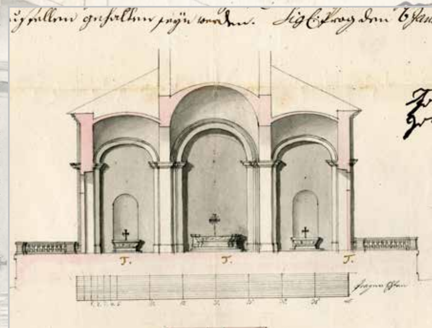
Nerealizovaný návrh: příčný řez svatohorským kostelem
